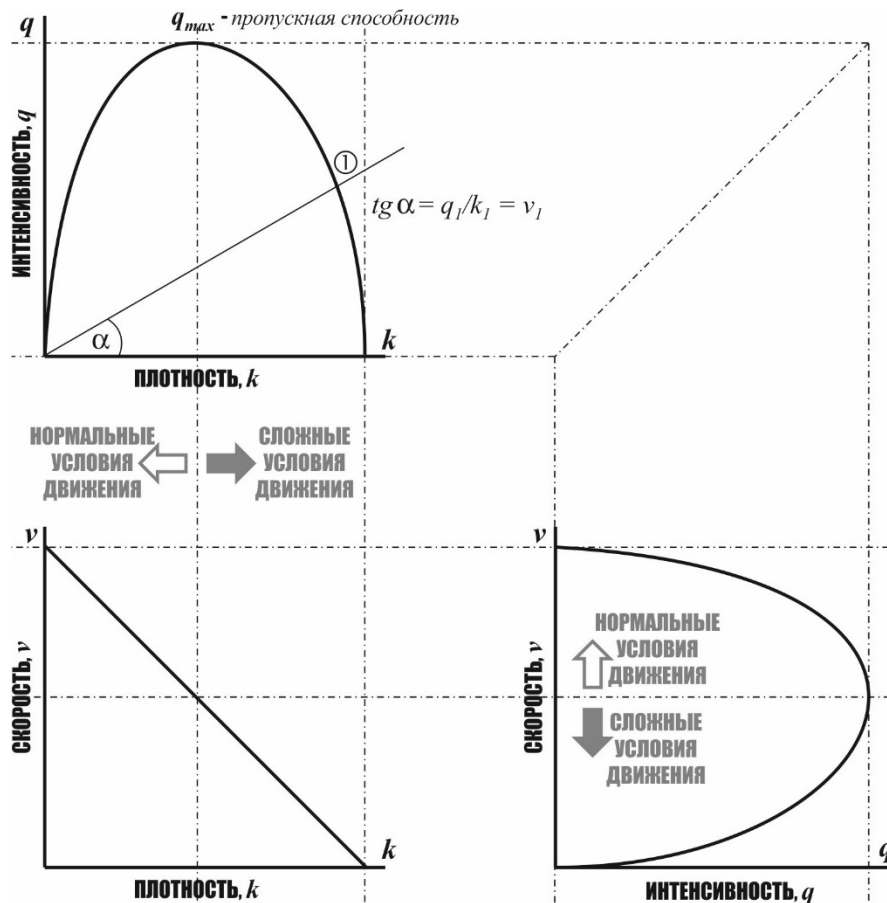
Рисунок 6.1.1 Зависимости между интенсивностью, плотностью и скоростью.
